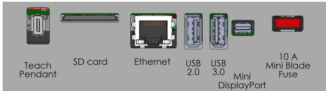
Externa anslutningsportar.
